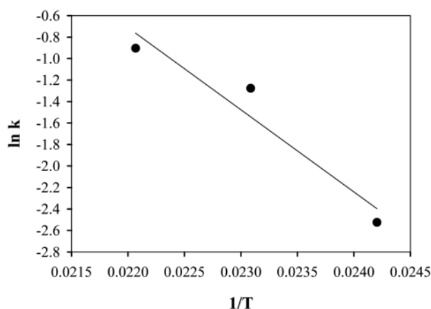
Fig. 2. Arrhenius plot.
